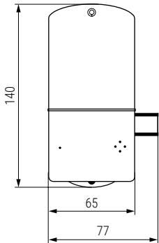
Cerradura Lock
