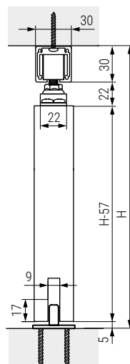
Aplicación con perfil al techo Application with profile for ceiling
