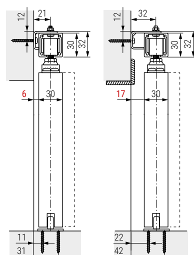
Aplicación con perfil y escuadra a la pared Application with profile and bracket for wall
