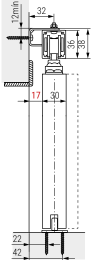
Aplicación con perfil y escuadra a la pared Application with profile and bracket for wall
