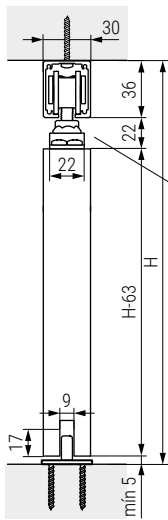
Aplicación con perfil al techo Application with profile for ceiling
