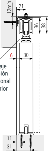
Aplicación con perfil y escuadra a la pared Application with profile and bracket for wall
