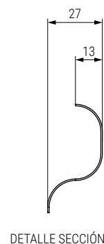
DETALLE SECCIÓN
