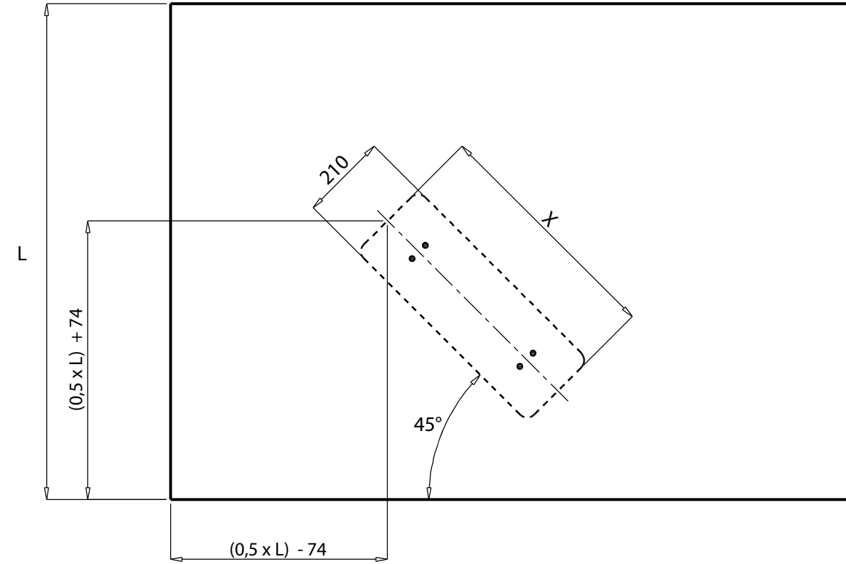
Dimensiones mínimas de corte en la parte fija de la placa rototraslante. Profundidad máxima del corte mm 24
