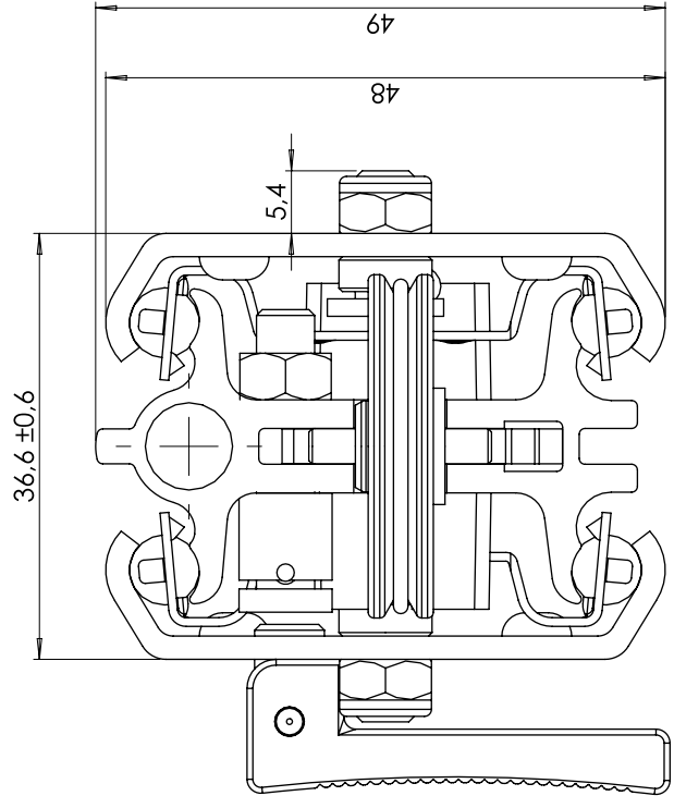
DETAIL A 2 : 1
