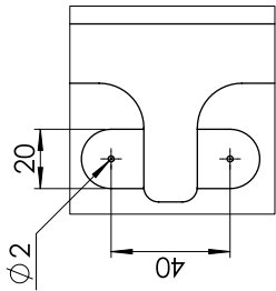
DETAIL G MAßSTAB 1 : 2
