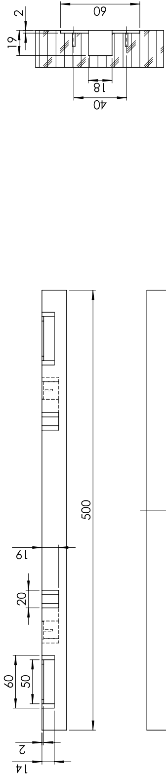
SCHNITT F-F MAßSTAB 1 : 2
