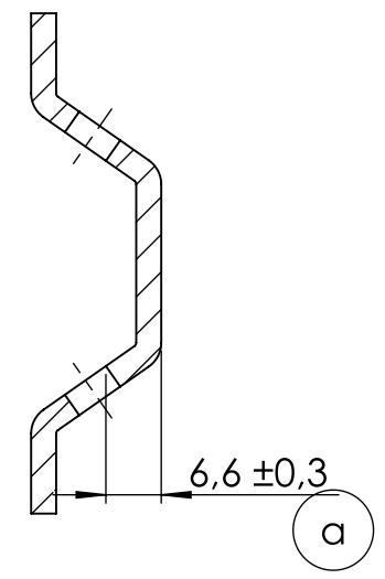
SCHNITT C-C MAßSTAB 1 : 1
