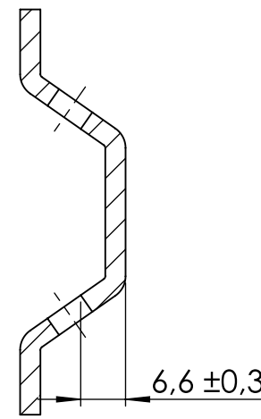
SCHNITT C-C MAßSTAB 1 : 1
