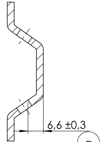
SCHNITT C-C MAßSTAB 1 : 1
