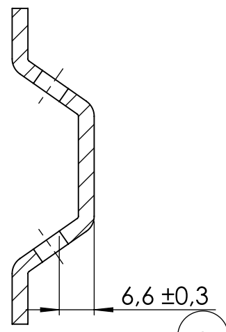
SCHNITT C-C MAßSTAB 1 : 1
