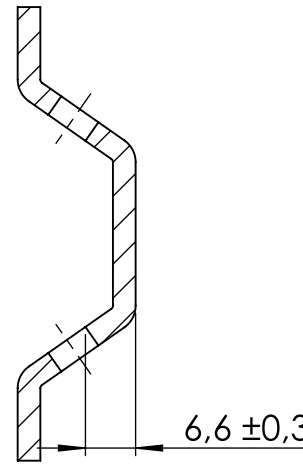
SCHNITT C-C MAßSTAB 1 : 1
