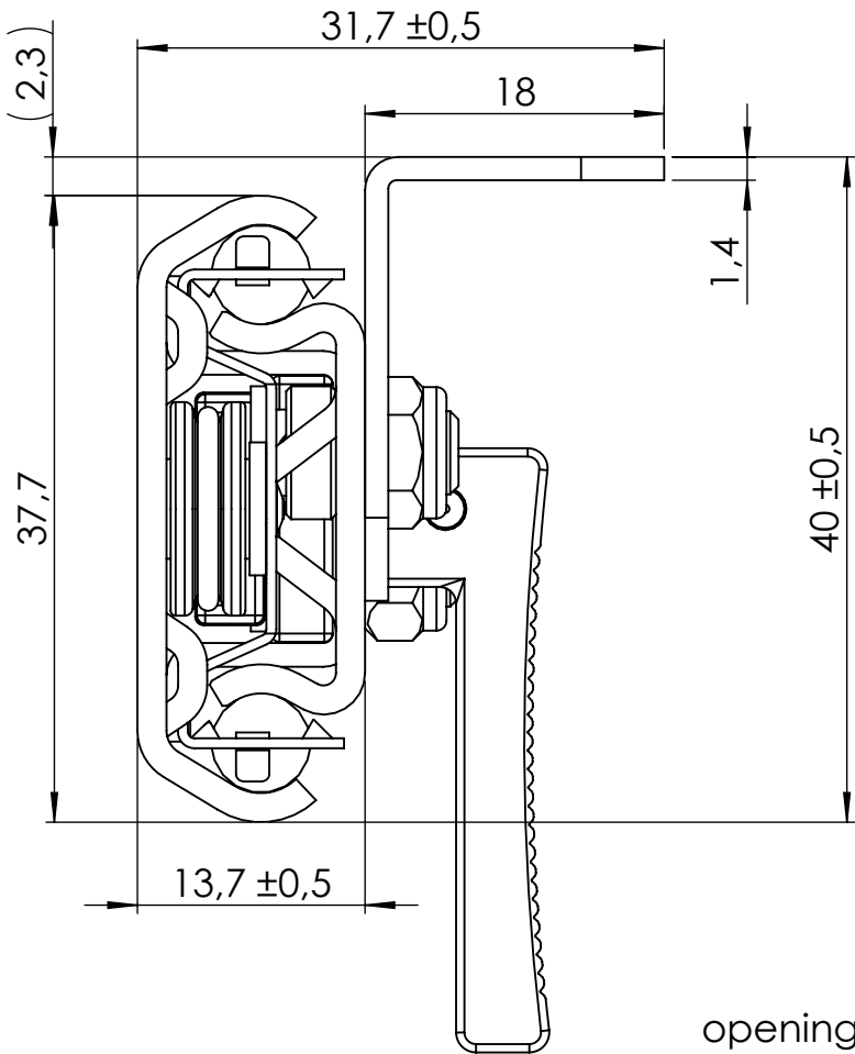
DETAIL A 2 : 1
