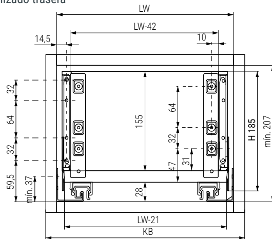
Mecanizado trasera
