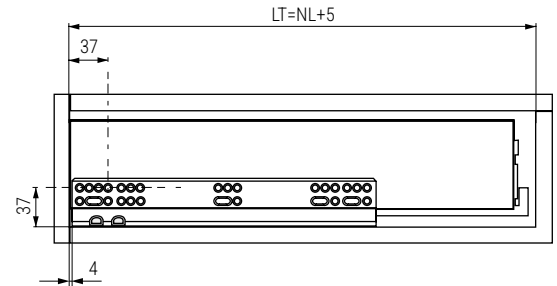
Mecanizado frente
