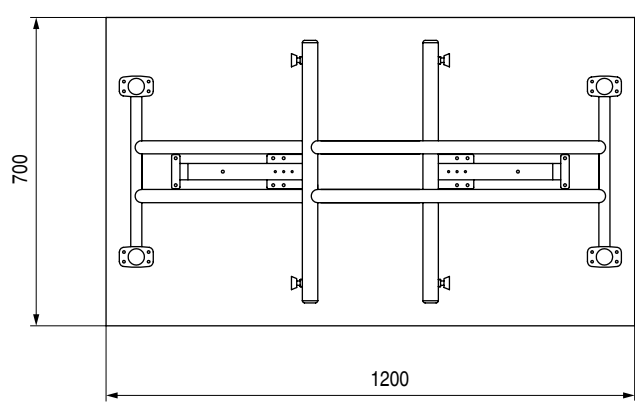
Medidas mínimas del tablero
