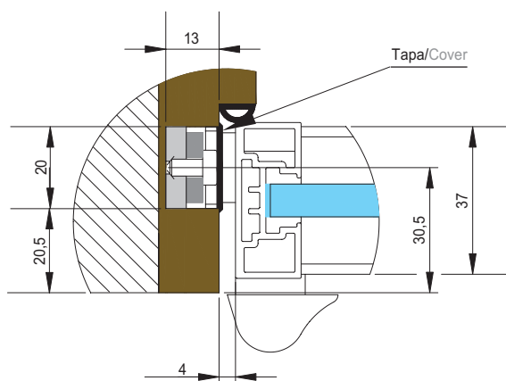
Mecanizado cerradero "Marco metálico" "Metal frame" striker machining
