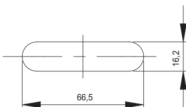
Mecanizado cerradero "Marco metálico" "Metal frame" striker machining
