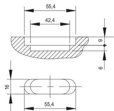
Mecanizado cerradero "Marco madera" "Wood frame" striker machining
