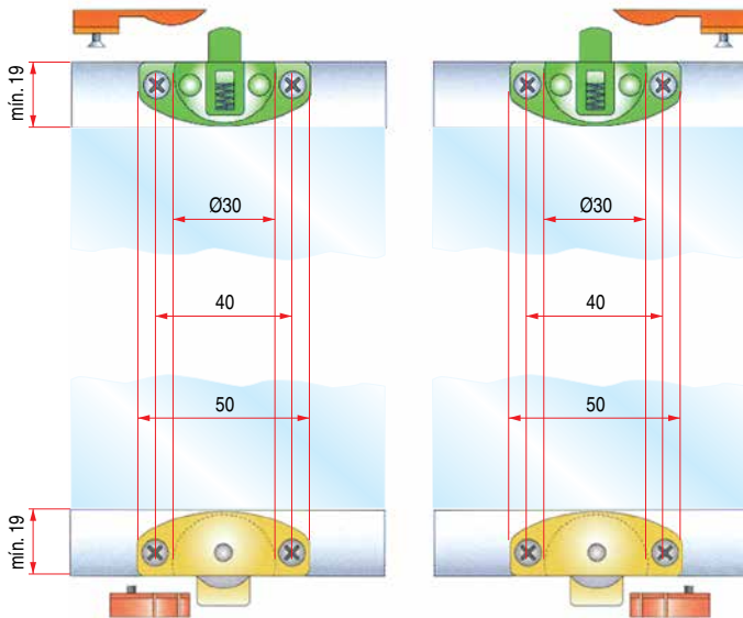
MINIBASE APLICADO A PUERTA DE ALUMINIO
