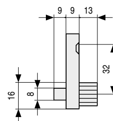
Soporte con tetón
