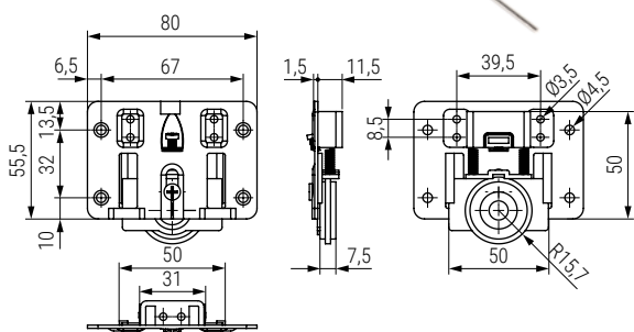
Carro inferior
