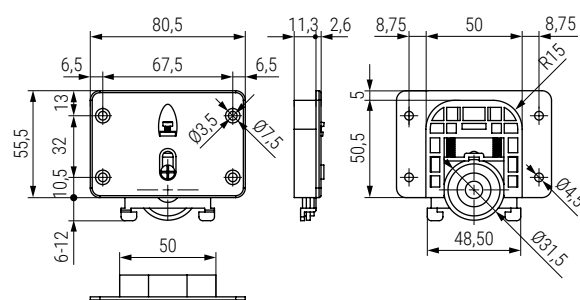
Carro inferior
