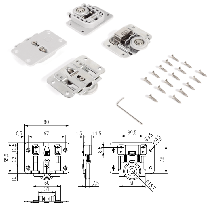
Carro inferior
