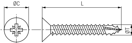
Pozidriv
