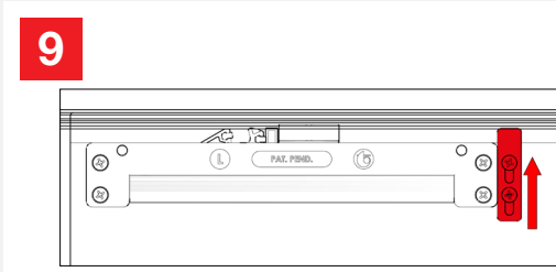
Activation Anti-Jumping/Attivazione Antisganciamento
