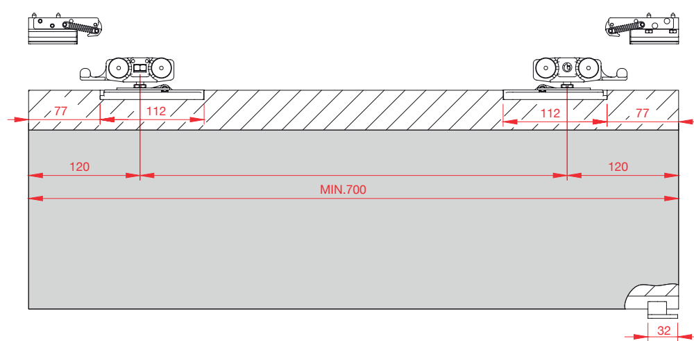
N.2 Hydraulic stopper N.2 Fermi idraulici
