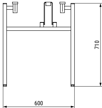
Dimensiones mínimas del Tablero Minimum table dimension
