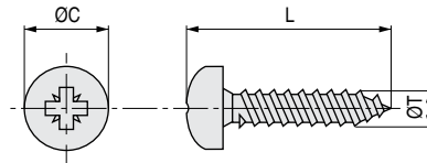
Pozidriv
