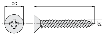
Pozidriv PZ2
