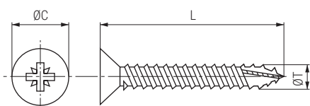
Pozidriv
